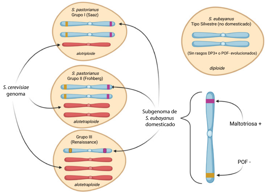
FIG. 2: Estructura genómica comparativa de los linajes de cepas lager del Grupo I (Saaz), Grupo II (Frohberg) y Grupo III (Renaissance).
